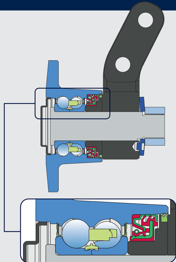
LIMENI POKLOPAC + RS ZAPTIVKA / RS ZAPTIVKA + KASETNA ZAPTIVKA + DVOUSNA ZAPTIVKA + KOVANI POKLOPAC
