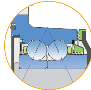
Limeni poklopac + RS zaptivka/ Trousna zaptivka + Čeona trousna zaptivka + Čelični poklopac
