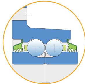
Trousna zaptivka / Trousna zaptivka
