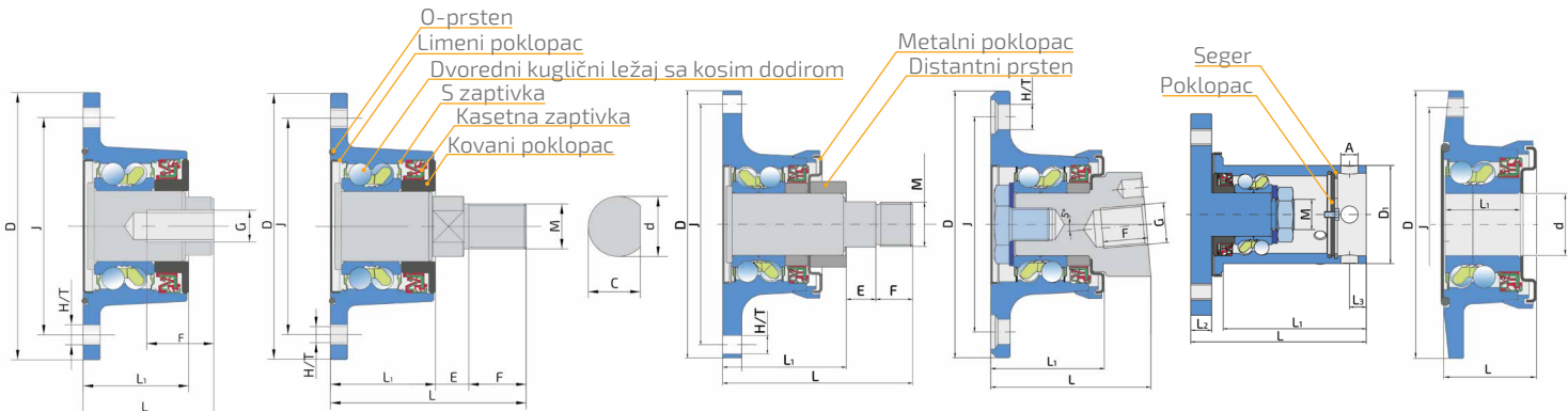
Slika 1 C= 75.86 kN *C= 66.35 kN Co=66.2 kN Co=56.49 kN Slika 2 C= 75.86 kN Co=66.2 kN Slika 3 C= 75.86 kN Co=66.2 kN Slika 4 C= 75.86 kN Co=66.2 kN Slika 5 C= 75.86 kN Co=66.2 kN Slika 6 C= 66.35 kN Co=56.49 kN
