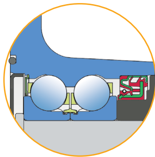
O-prsten + Limeni poklopac + RS zaptivka/Kasetna zaptivka + Kovani poklopac
