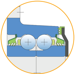
Trousna zaptivka/Trousna zap- tivka+ Čeona trousna zaptivka + Čelični poklopac
