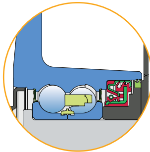
Limeni poklopac + RS zaptivka/RS zaptivka + Kasetna zaptivka + Dvousna zaptivka + Kovani poklopac
