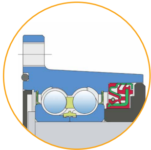
O-prsten + Limeni poklopac + RS zaptivka/RS zaptivka + Kasetna zaptivka + Kovani poklopac
