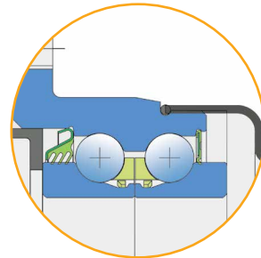
Plastični poklopac + Trouсна zaptivka/ RS zaptivka + Navojna metalna kapa
