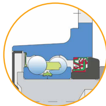
Limeni poklopac + RS zaptivka/Kasetna zaptivka + Kovani poklopac
